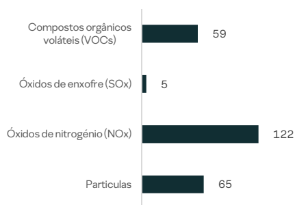
EMISSIONES ATMOSFÉRICAS (TON)
